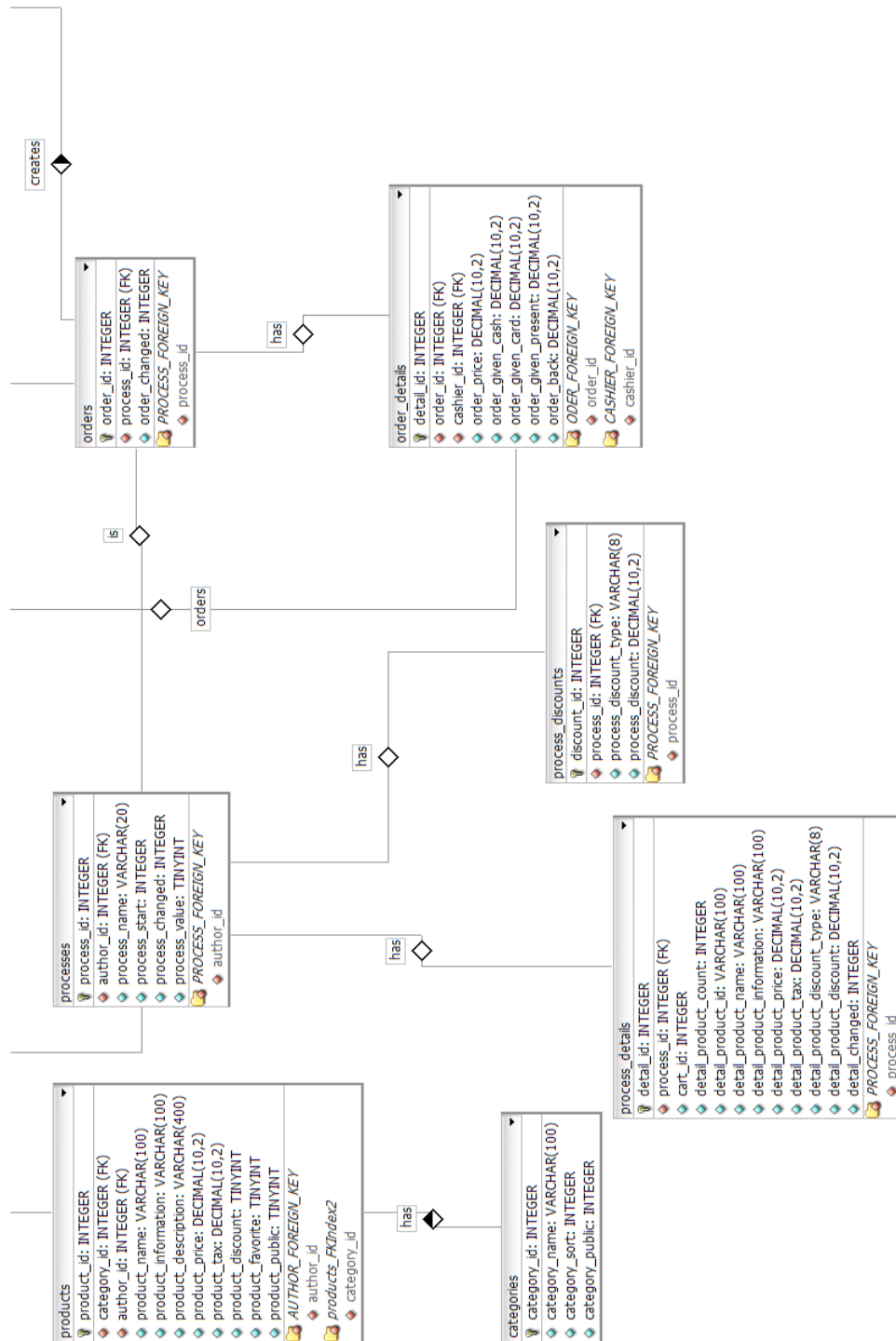
Abbildung C.2: Datenbankschema 2 von 2
